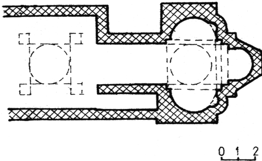
Пл. 10. Св. Арханѓели, манастир Св. Наум (цртеж: Мирка Илоска).
