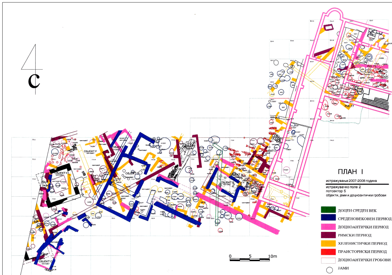
Пл. 9. Остатоките од Светиклиментовите манастирски конаци (објект D, простории 1 – 6а) (дигитал.: Горан Панчев).
