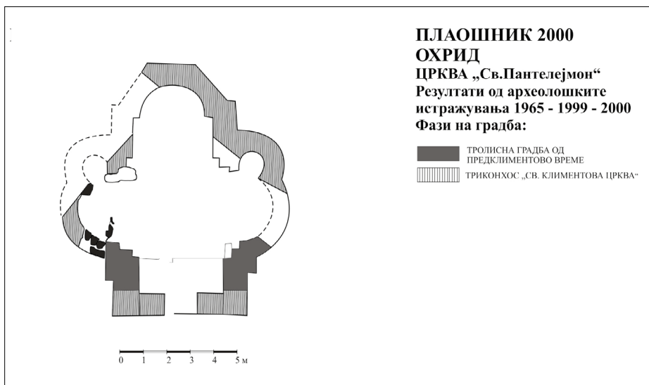
Пл. 3. Основа на триконхосот по обновата од Св. Климент (цртеж: Тодор и Тања Паскали).
