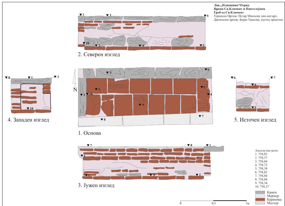
Цртеж 1. Светиклиментовиот гроб во црквата на Плаошник (Петр Мисоски; дигитал.: Бојан Танески).
