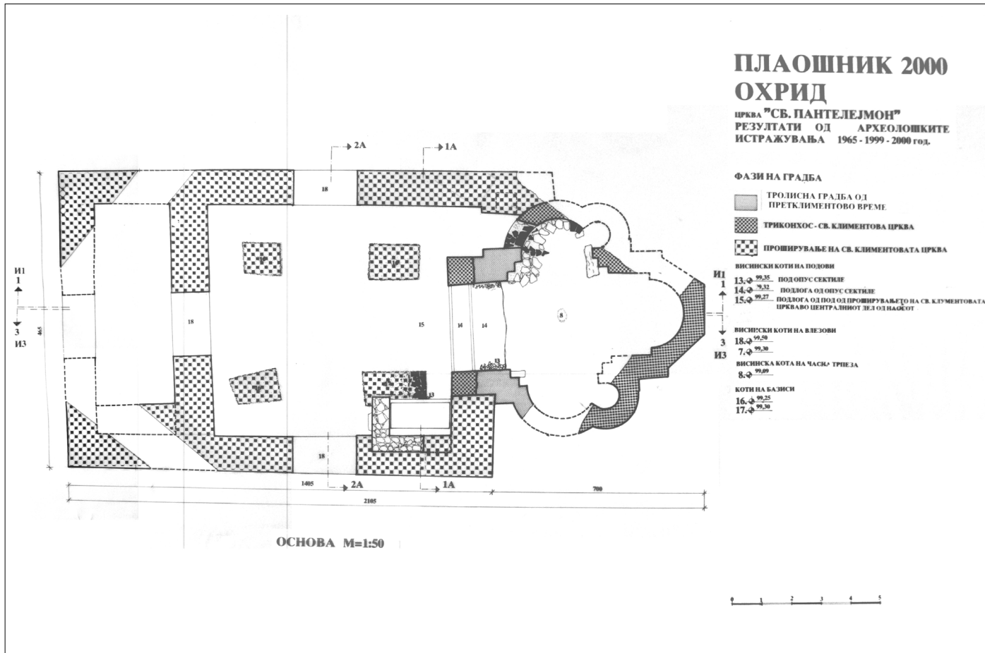
Пл. 4. Проширување на триконхосот кон запад во времето на Св. Климент (цртеж: Тодор и Тања Паскали).
