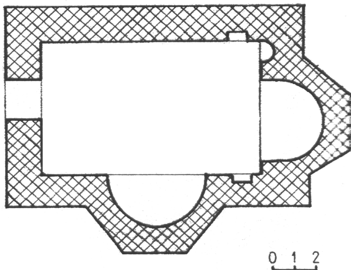
Пл. 13. Издеглавје, Охридско, Св. Никола, основа на двоконхална црква (цртеж: Мирка Илоска).
