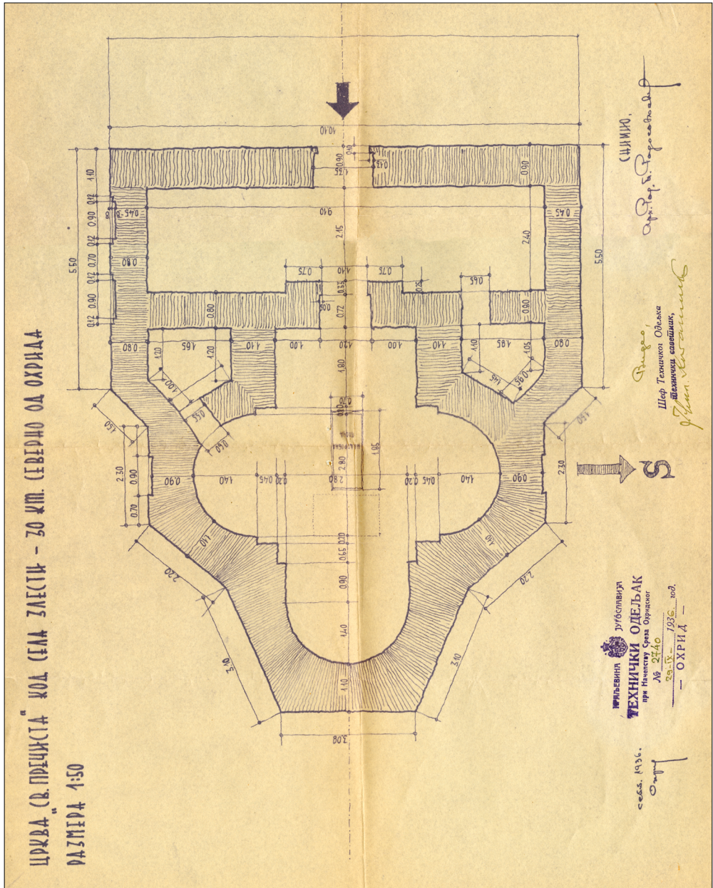
Пл. 12. Злести, Охридско, основа на триконхална црква (П. Радосављевић). Народен музеј во Белград, Заоставштина на Милан Кашанин, Архивска кутија, бр. 2, 1/18/6.
