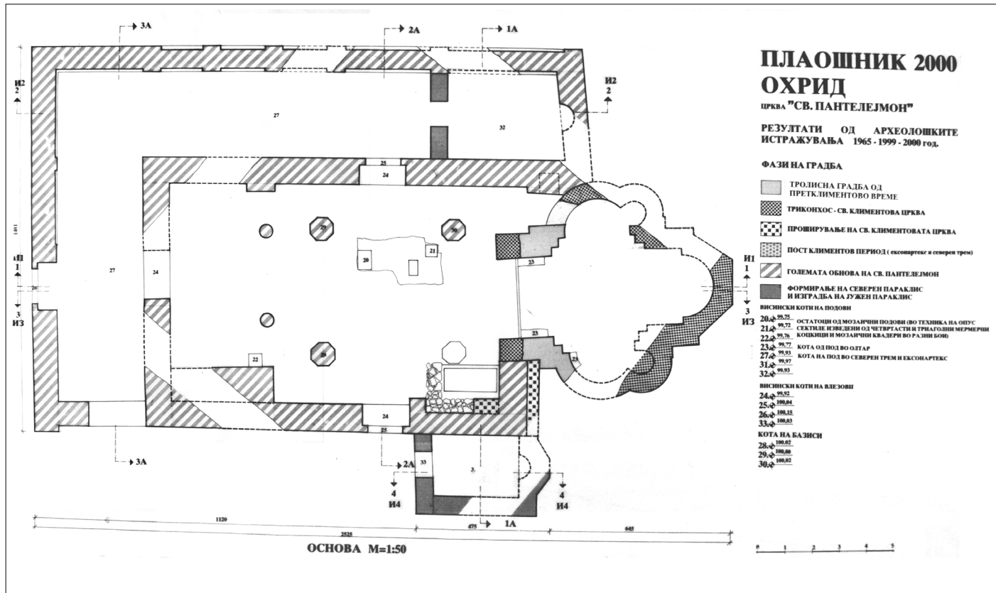
Пл. 5. Светиклиментовата црква по проширувањето во XIV–XV век (цртеж: Тодор и Тања Паскали).
